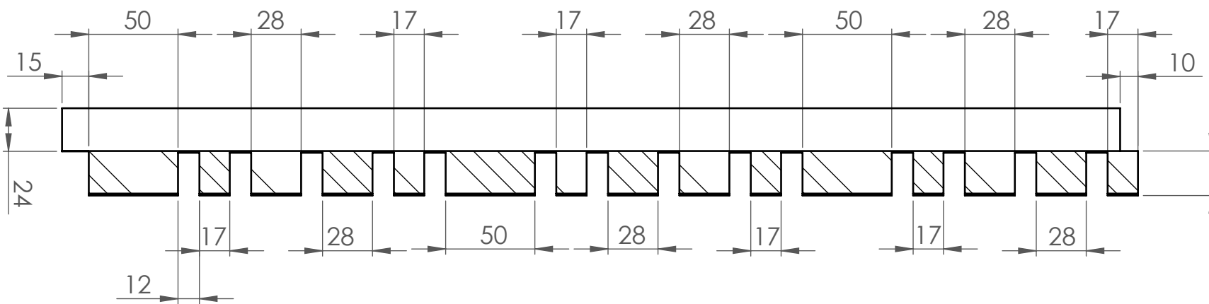
B-B (1 : 3)
